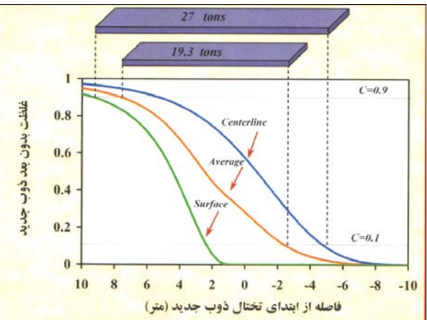
پیش بینی مقدار روزن تختال مخلوط شده با معیارهای مختلف انتخاب
