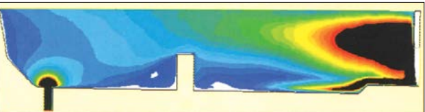
شکل ۱: الگوی جریان مذاب در تاندیش
