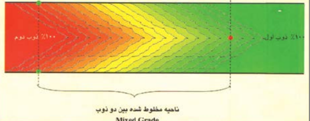
شکل ۲: الگوی اختلاط (Intermixing) در ناحیه بین دو ذوب مخلوط شده در تختال منجمد شده
