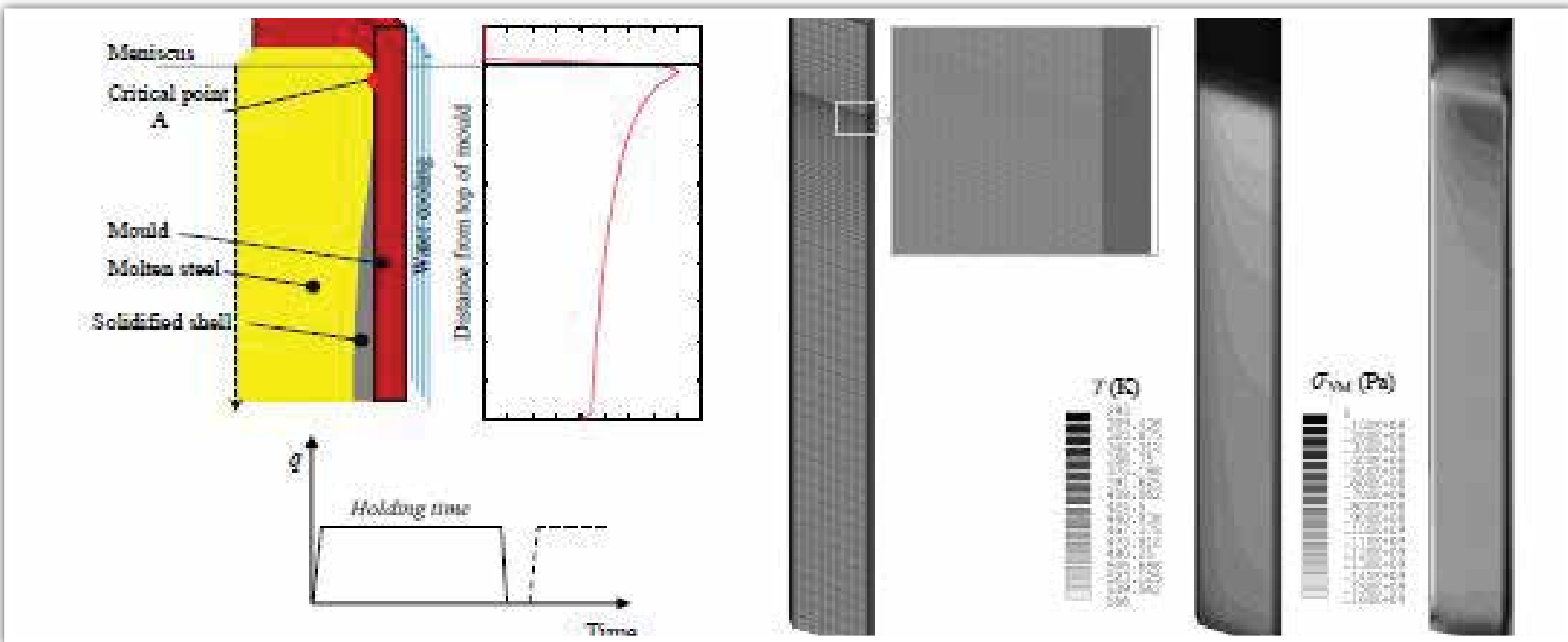
شکل ۴. هندسه قالب و توزیع تنش و حرارت در قالب های مسی آبگرد ریخته گری مداوم
