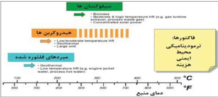
شکل ۱. انواع مایع های مورد استفاده در محدوده کاری سیستم ORC.
