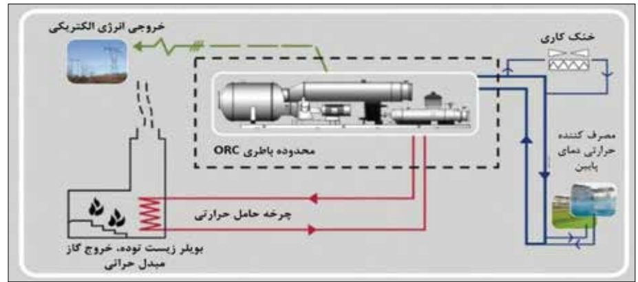
شکل ۲. حلقه حامل حرارتی.
