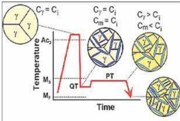
شکل ۲- شمایتمیک عملیات حرارتی تولید فولاد Q&P.
