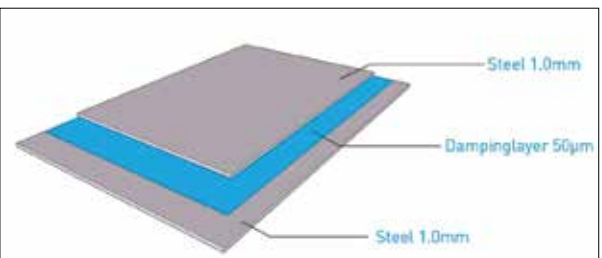
شکل ۱- ساختار شمشیک ورق‌های فولاد بدون صدا
