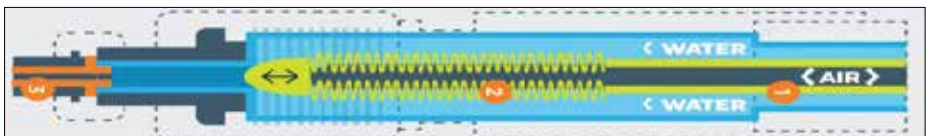
شکل ۳ - شماتیکی از ساختار نازل‌های خنک‌کاری ثانویه DynaJet Flex تولیدی شرکت پریمتالز
