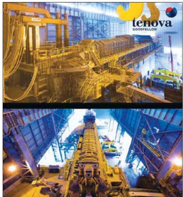
شکل ۴- سیستم پیش گرمایش مواد ورودی به کوره قوس الکتریکی، پیشنهاد شده توسط شرکت Tenova
