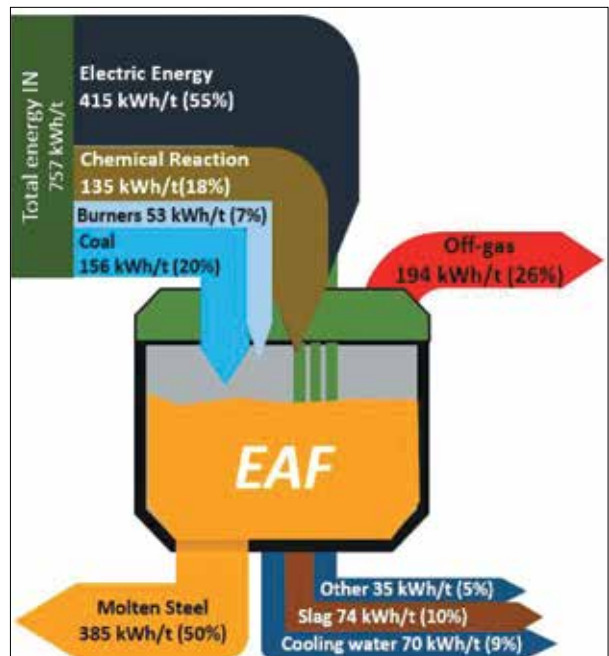
شکل ۱- موازنه انرژی در کوره قوس الکتریکی
