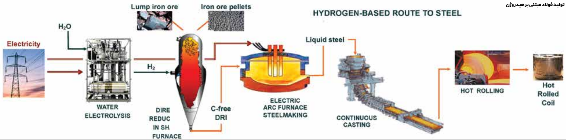
تولید فولاد مبتنی بر هیدروژن
