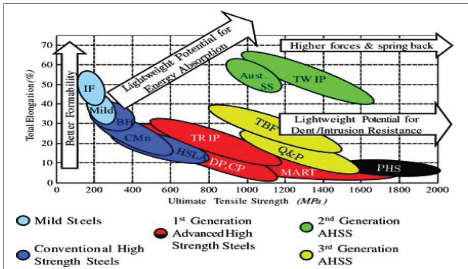
شکل ۱- روند توسعه فولادهای AHSS.
