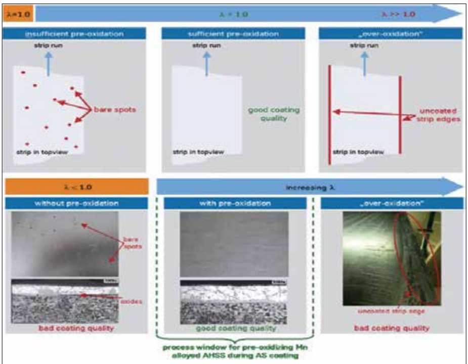
شکل ۲- اهمیت پارامتر در عملیات پیش‌اکسیداسیون برای آلومینایزینگ فولاد AHSS.
