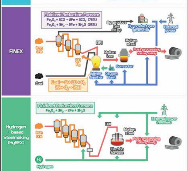
مقایسه فرایندهای کوره بلند با فرایند FINEX و فرایند بر پایه هیدروژن در POSCO
